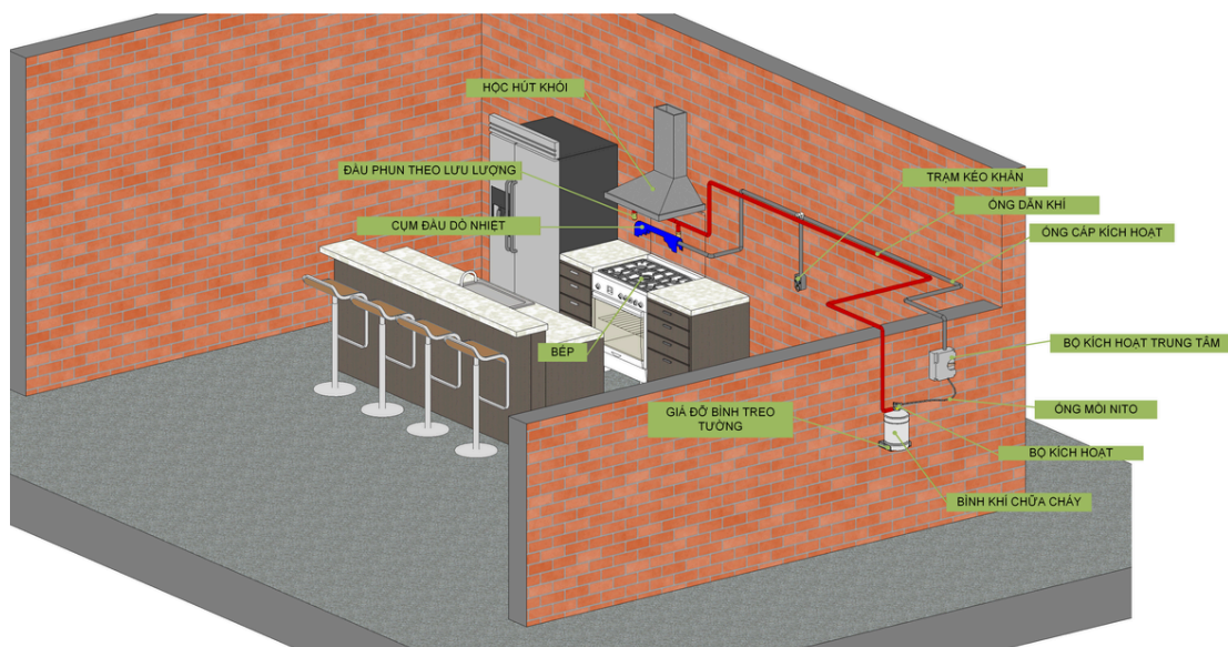
HỆ THỐNG CHỮA CHÁY bếp whdr/ WHDR KITCHEN FIRE SUPPRESSION SYSTEM
