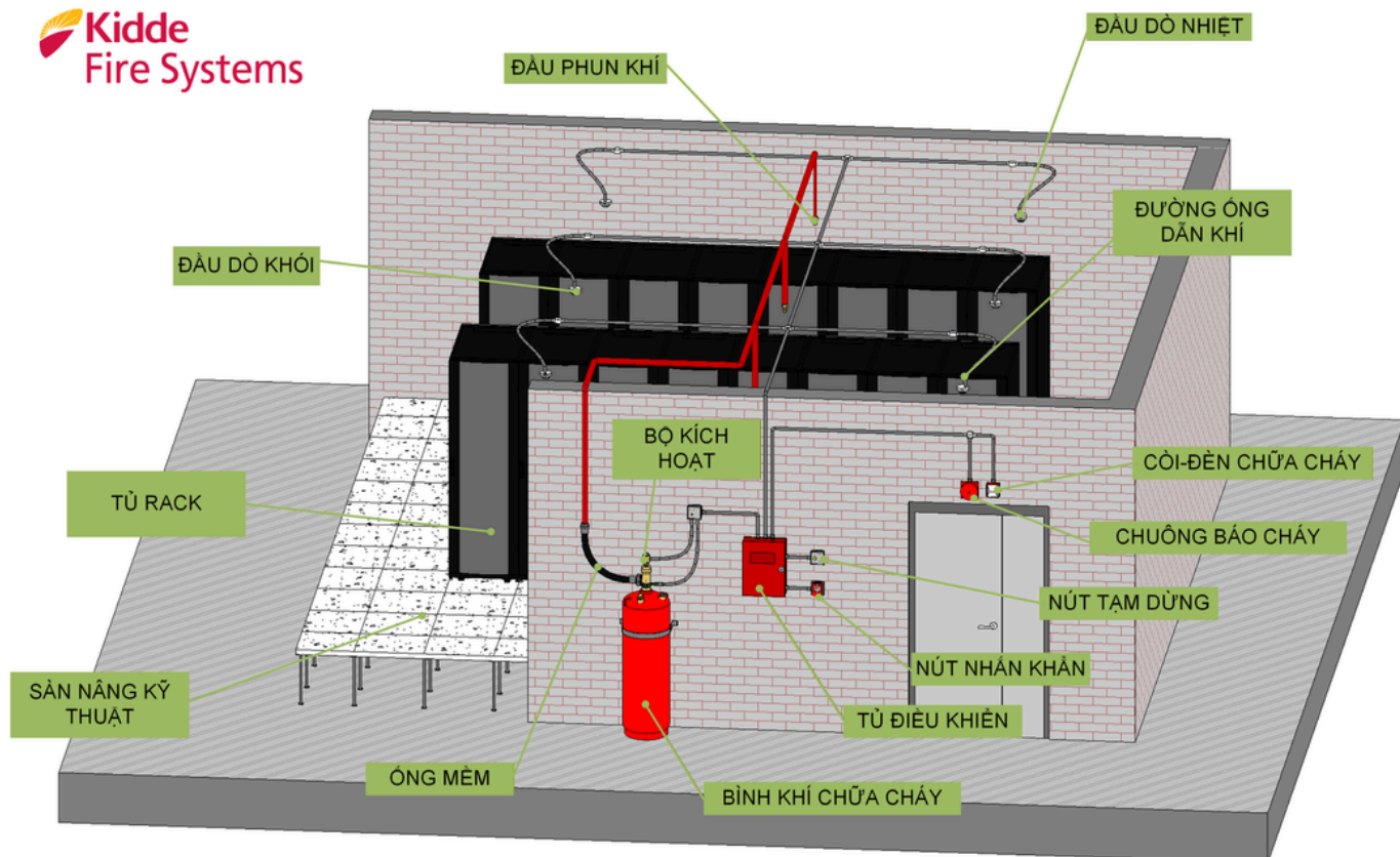
HỆ THỐNG CHỮA CHÁY FM200/ FLUORO-K / FM-200 / FLUORO-K FIRE SUPPRESSION SYSTEM
